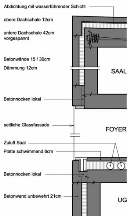
Querschnitt durch die zweischalige Gebäudehülle.
